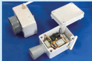
無線通信技術を活用した河川水位計
